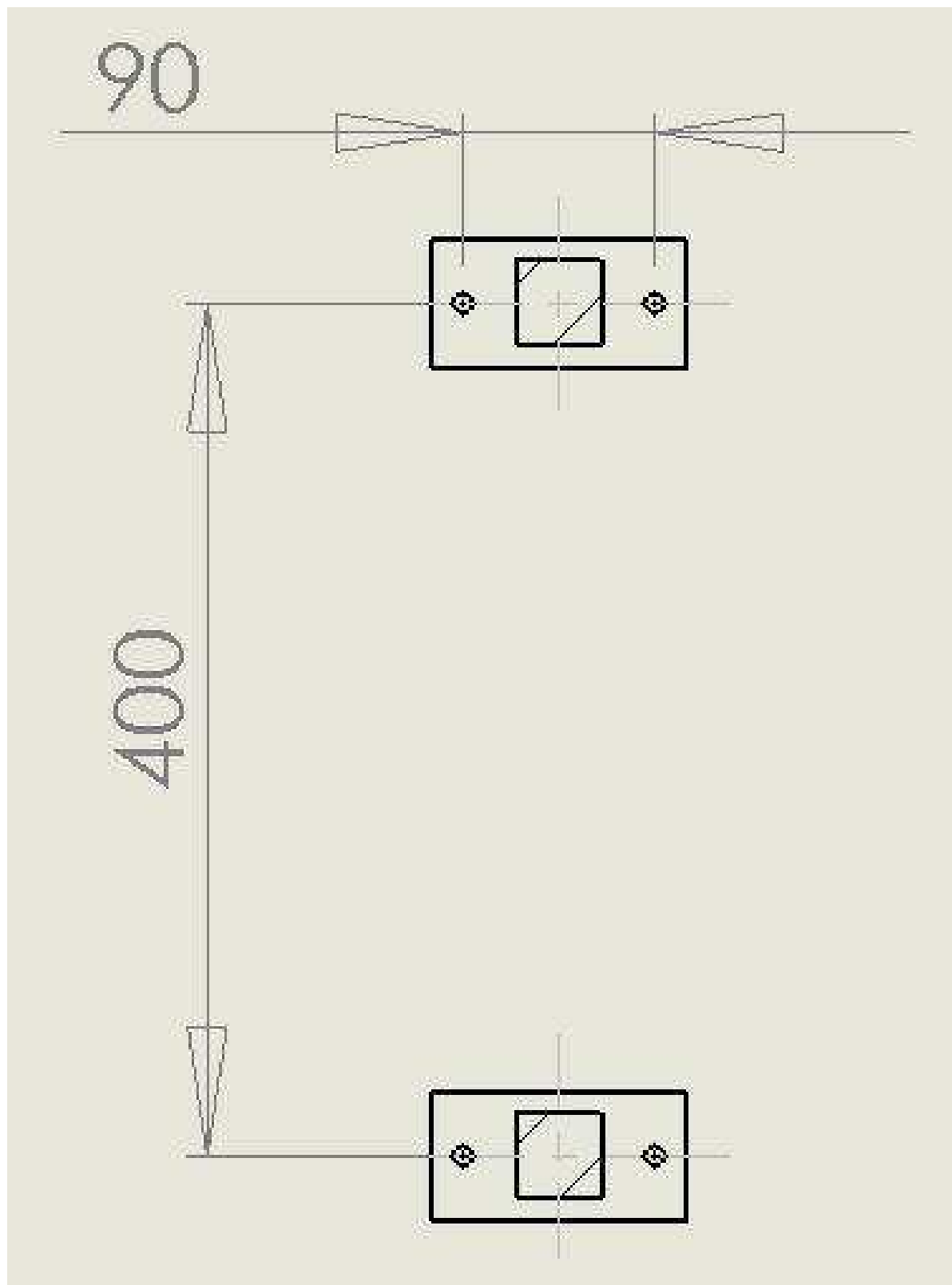
Skizze Bohrbild bei Wandmontage
